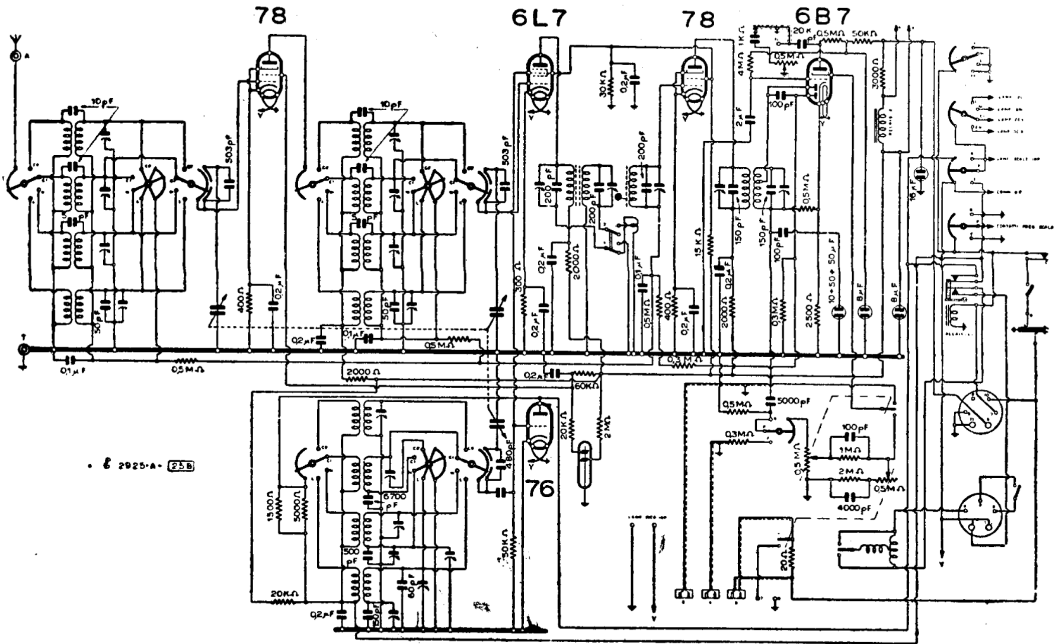
Schema elettrico, escluso l'alimentatore, del radiotelegrafo Salar mod. « 948 ».
